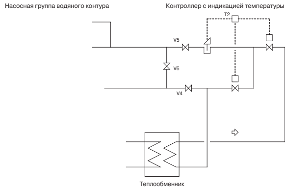
Принципиальная схема для части В (трехходовой клапан → двухходовой клапан)
